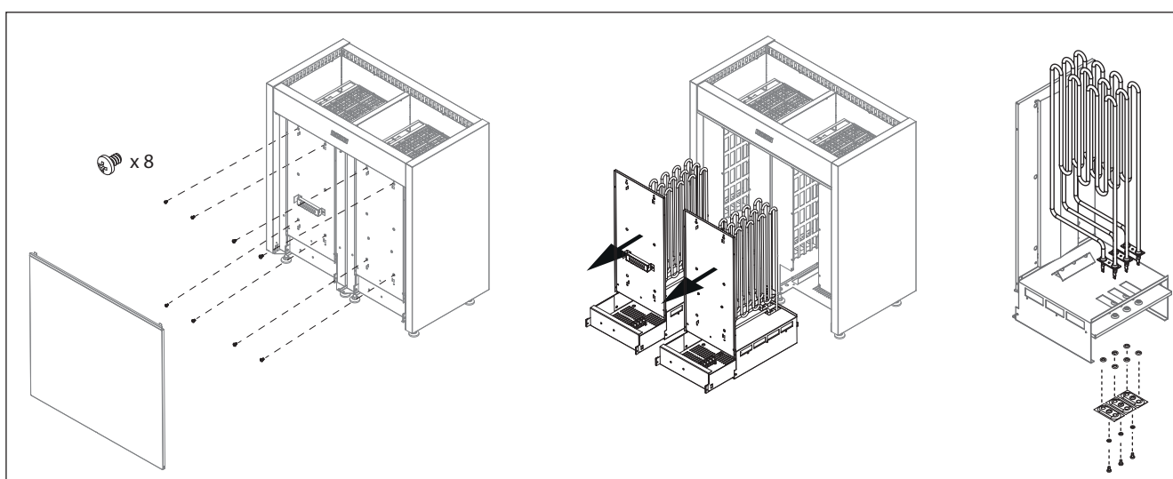
Figure 8. Remplacement des éléments de résistance.
