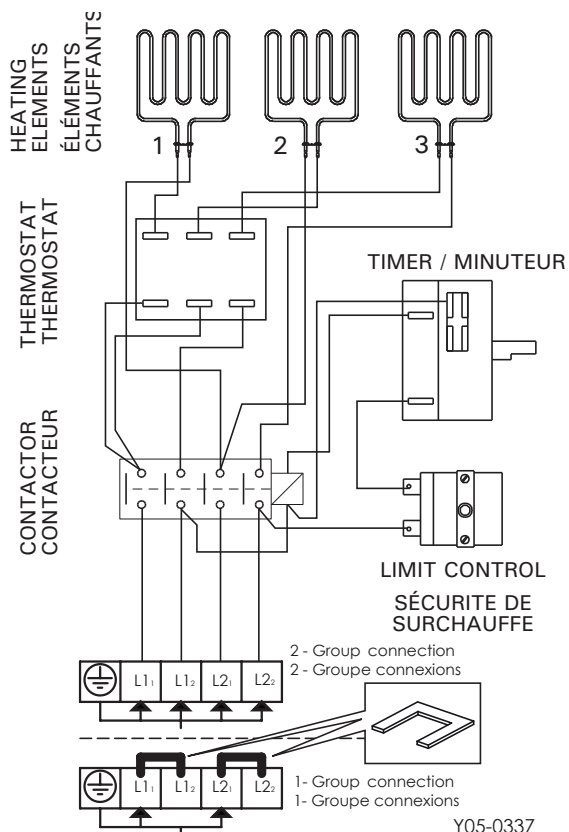
Figure 5. Connexions électriques de poêle.
